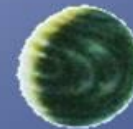
ПЛУТОН
