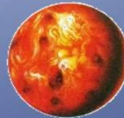
МАРС
