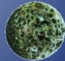
МЕРКУРИЙ
